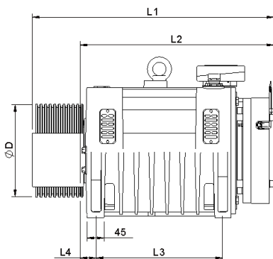
Rolle Ø160/Ø240/Ø270
